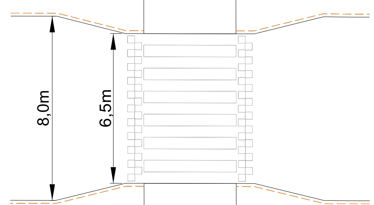
TYYPPIPOIKKILEIKKAUS, 1:100 KOROTETTU SUOJATIE 0.81 4.90 0.90 +0.08 +0.00 +0.08 Lumattava reunakivi 80 mm PÄÄLLYSTIEN YLAOSA Ab 16/120 8 cm PÄÄLLYSTIEN ALAOSA Tai SRM 0-65...100 8 cm YHTEENSÄ Mitoitusnopeus hidasteen kohdalla Henkilöauto 30 km/h Raskas ajoneuvo 10 km/h
