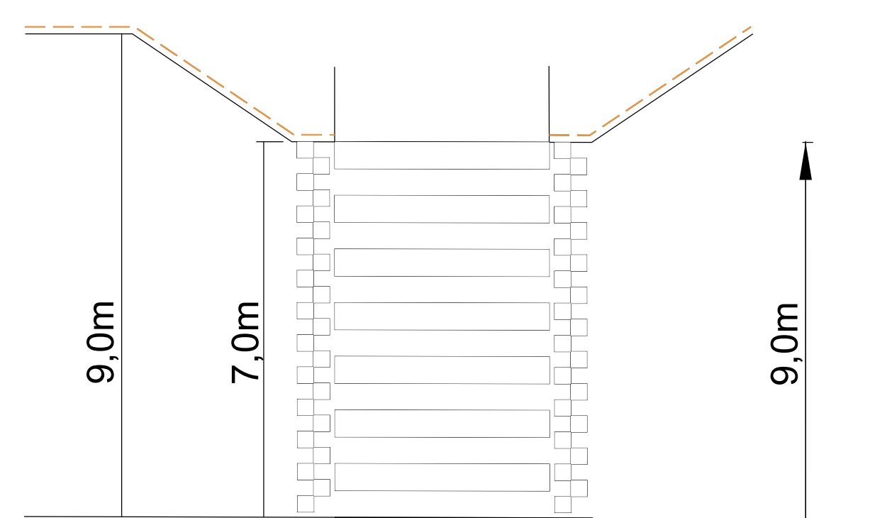
TASOKUVA, 1:100 SUOJATIENTÄN KAVENNUS JA KOROTETTU SUOJATIE, KOULUKATU
